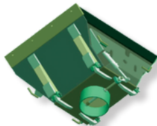
Sortie Ronde Ø 285mm Round outlet
